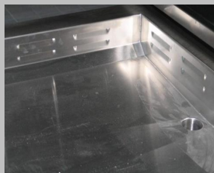
Seiten-Abluftsystem für gleichmäßige Ab- saugung über den gesamten Körperbereich. Der Boden ist vollkommen glatt und sehr gut zu reinigen. Das Eindringen von Wasser oder Schmutz wird verhindert.
